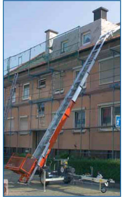
Bauaufzüge
